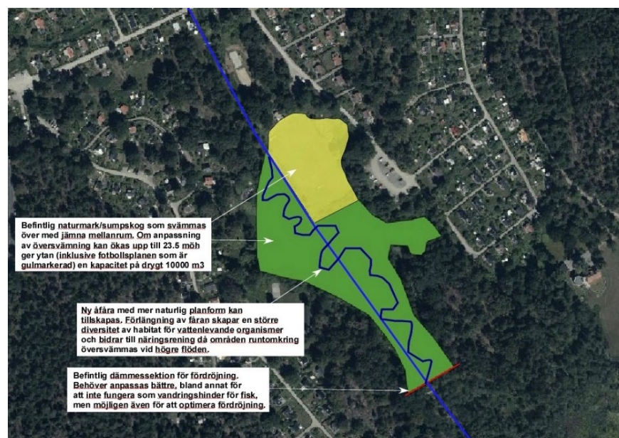
Figur 9. Principskiss över åtgärd i nedre Flatendiket. Grönmarkerad yta är befintlig sumpskog/översvämningsyta, gulmarkerad yta är låglänt yta där det idag ligger en fotbollsplan. Figur från DHI (2018).
